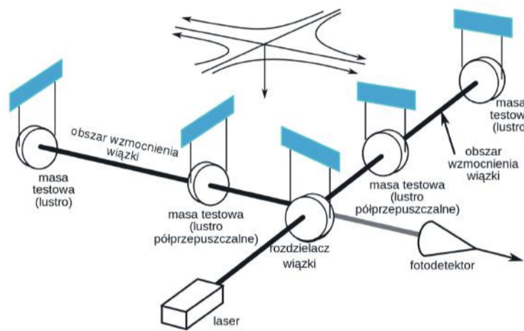
Schemat działania interferometru laserowego – Grafika LIGO
