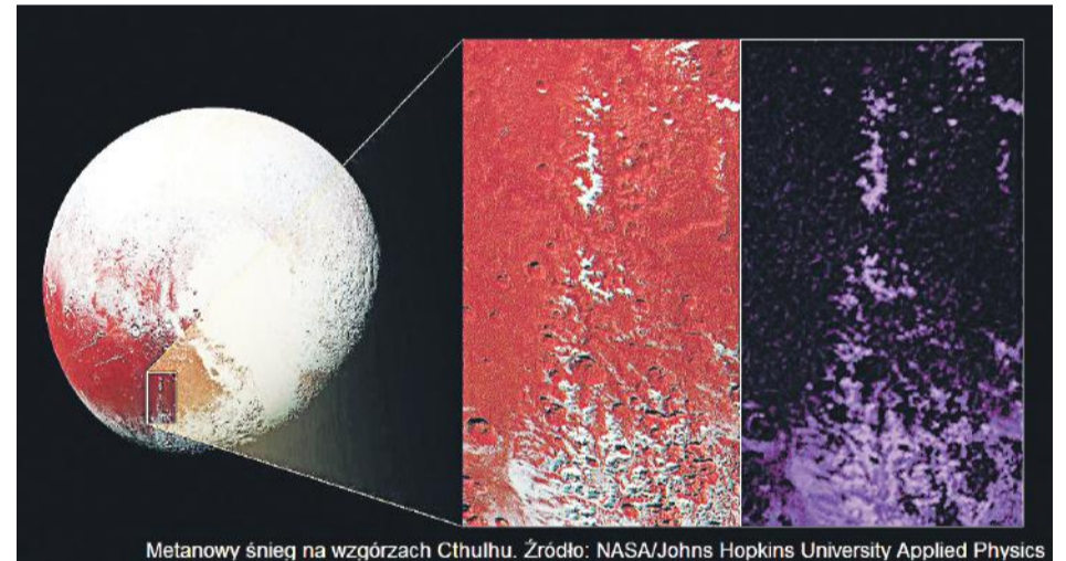
Metanowy śnieg na wzgórzach Cthulhu. Źródło: NASA/Johns Hopkins University Applied Physics
