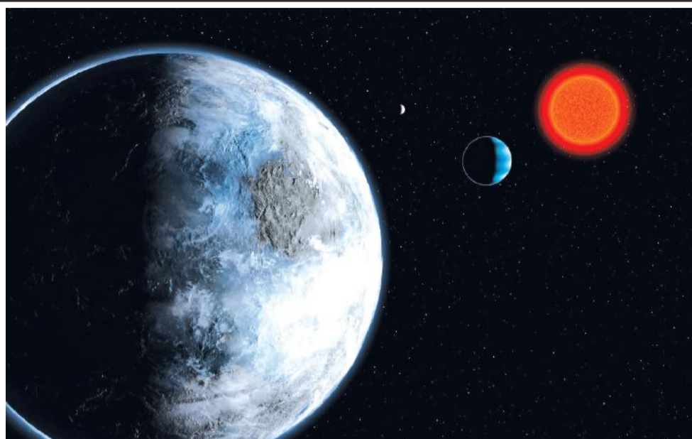
Artystyczna wizja układu planetarnego wokół gwiazdy Gliese 581
