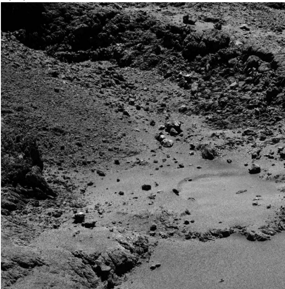
Zdjęcie powierzchni komety 67P/Churyumov-Gerasimenko wykonane w dniu 11 maja 2016 kamerą wąskokątną OSIRIS. Rosetta była wtedy oddalona od komety o 9,9 km. Skala zdjęcia to 0,16 m/piksel. Źródło: ESA/Rosetta/MPS for OSIRIS Team MPS/UPD/LAM/IAA/SSO/INTA/UPM/DASP/IDA
